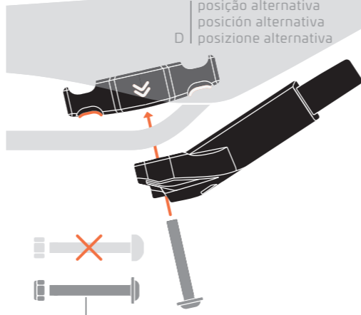
usar parafuso originalis utilizar tornillo originales usa vite originali E
